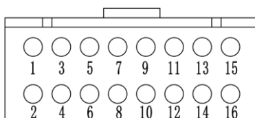
图 2-3 CN3 管脚（母座）
