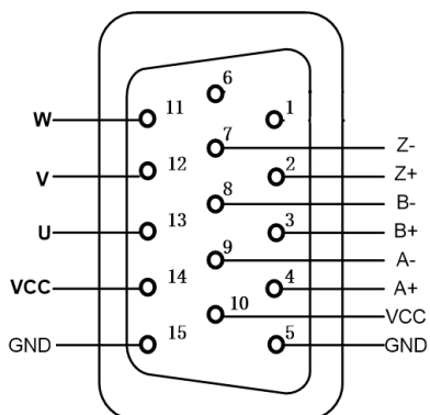
图 2-4 伺服电机编码器接口的管脚定义
