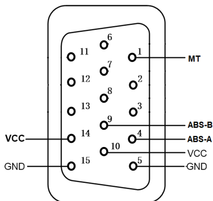
图 2-6 绝对值电机编码器接口定义
